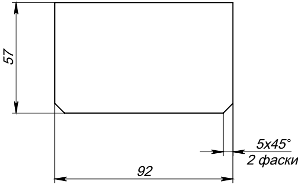
Поз.2 (Ребро)
